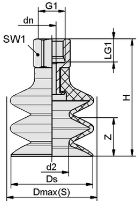
设计参数 FSG 20 NBR-ESD-55 G1/8-IG
