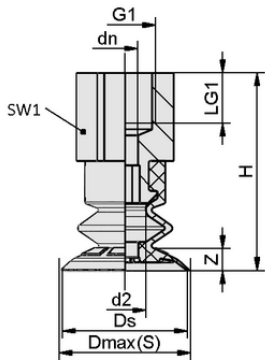
设计参数 SFB1 40 EPDM-45 G1/4-IG
