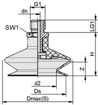
设计参数 FSGA 16 NBR-ESD-55 M5-AG
