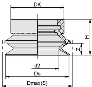
设计参数 BCG 50 NBR-ESD-55 SC095
