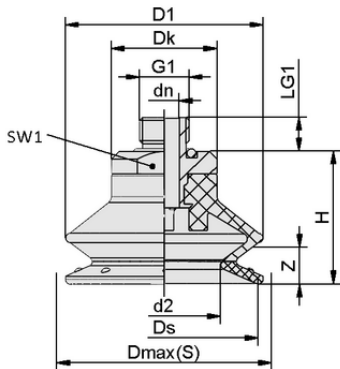
Design data SDC1 60 PU 30/60 G3/8-AG
