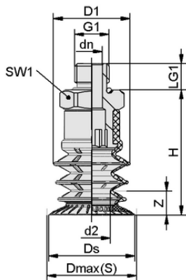
设计参数 PSPF 53 SI-30/55 G3/8-AG
