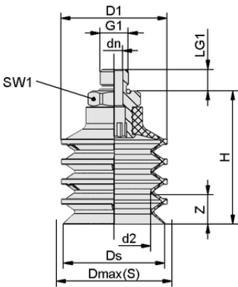
设计参数 FSGC 50 NBR-55 G3/8-AG
