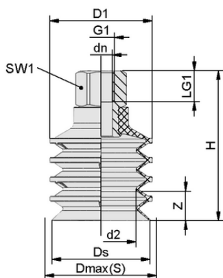
设计参数 FSGC 50 NBR-55 G3/8-IG
