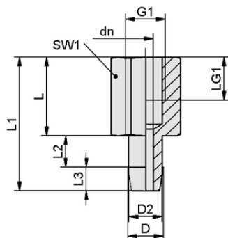
设计参数 SA-NIP N062 G1/8-IG DN350
