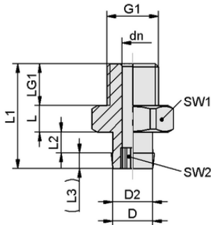
设计参数 SA-NIP N062 G1/8-AG DN350
