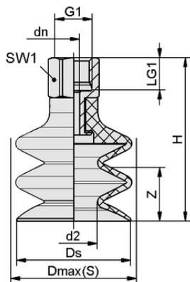
设计数据 FSG 32 SI-MD-55 G1/4-IG
