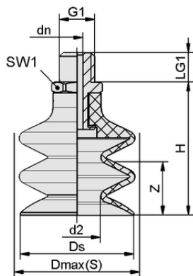
设计数据 FSG 42 SI-MD-55 G1/4-AG
