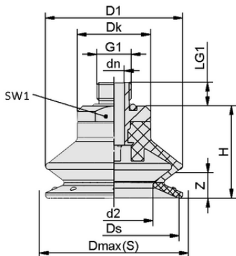
Design data SDC1 60 PU 30/60 G1/4-AG
