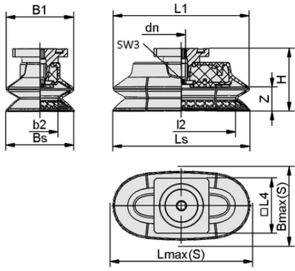
设计参数 SAOXB 40x20 ED-85 RA MOD
