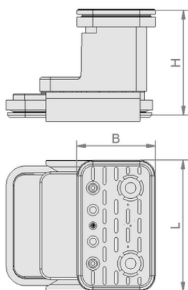
设计参数 VCBL-K2 120x50x100 Q
