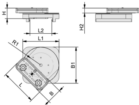
设计参数 VCBL-S1 120x50x32.7 D-360 TV
