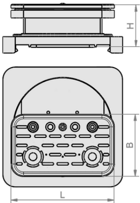
设计参数 VCBL-S1 125x75x32.7 D-360 TV
