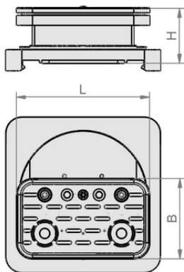
设计参数 VCBL-S4 125x75x50 D-360 TV
