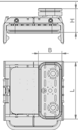
设计参数 VCBL-K1 125x75x85 L
