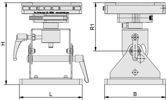
设计参数 VC-M 165x165x220.5
