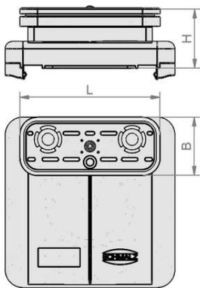
设计参数 VCBL-S1 120x50x32.7 TV
