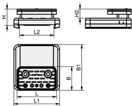
设计参数 VCBL-S4 125x75x50 TV
