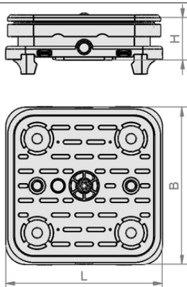
设计参数 VCBL-S1 120x120x32.7 TV-S
