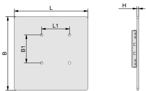
设计参数 ISAP-B 195x195x5
