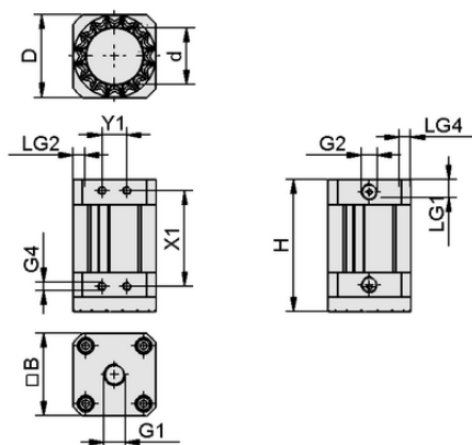
设计参数 SGM-SV 40 G1/4-IG
