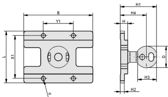
设计参数 HTS-A5 SGM-HP 40x121 OP
