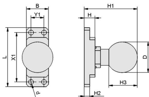
设计参数 HTS-A5 SGM-HP 50 OP
