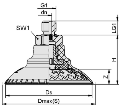
设计参数 SAXM 30 ED-85 M14x1.5-AG
