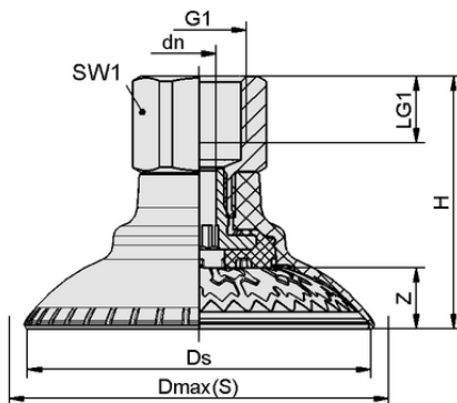
设计参数 SAXM 40 ED-85 G3/8-IG
