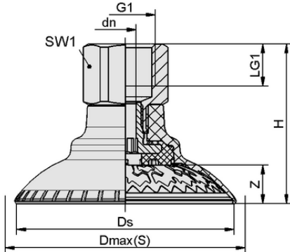
设计参数 SAXM 50 ED-85 G3/8-IG
