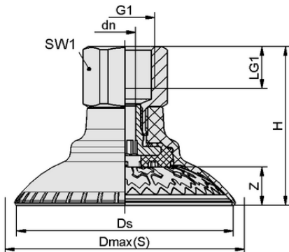
设计参数 SAXM 60 ED-85 G3/8-IG
