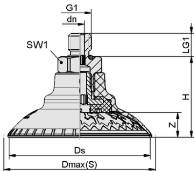
设计参数 SAXM 80 ED-85 M14x1.5-AG
