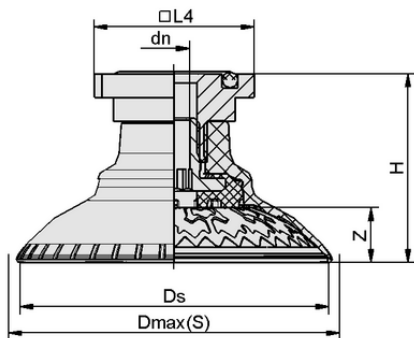
设计参数 SAXM 80 ED-85 RA
