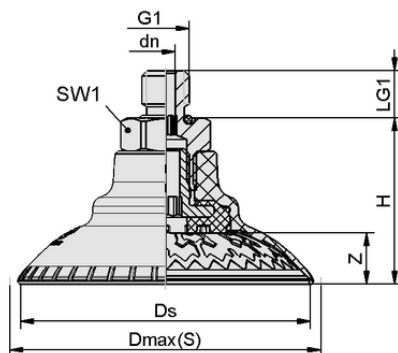
设计参数 SAXM 40 ED-85 G1/4-AG
