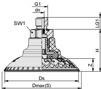
设计参数 SAXM 80 ED-85 G3/8-AG
