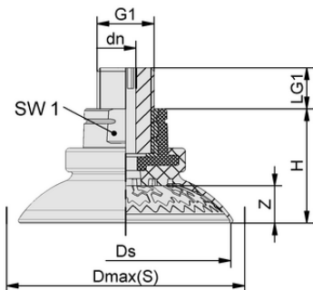
设计参数 SAX 115 ED-85 G1/4-AG RP
