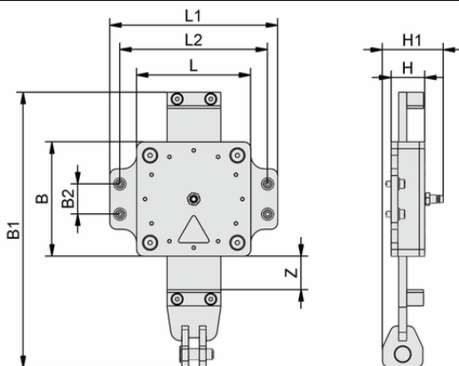
Design data FST-C 100-HD1
