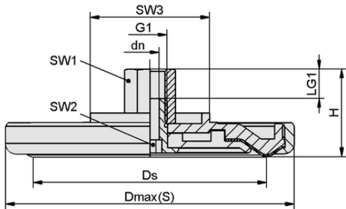
设计参数 SPL-HT 90 ST G1/4-IG
