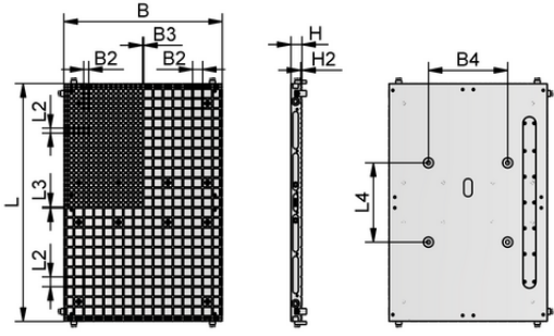
设计参数 MPL 400x300x28 12,5x12,5 3x3
