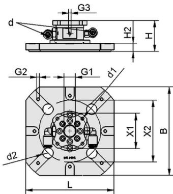
设计参数 SWGm-5A 115x115x40 1xE100 A PEEK
