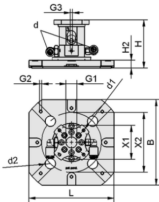
设计参数 SWGm-6S 146x146x65 1xE100 A PEEK
