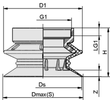
设计参数 SAUG-SCG 40 SI-HD-65
