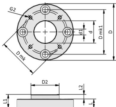
设计参数 FLAN-PL 63.5x10 AL-EL VEE
