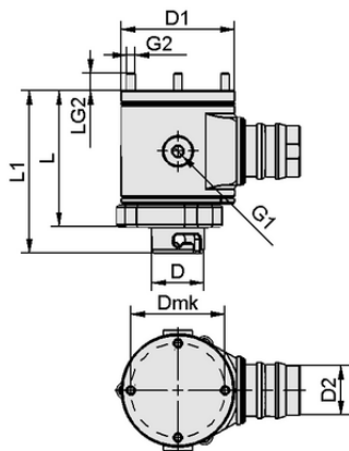
设计参数 VEE-RU 55x83.5 60 QCM
