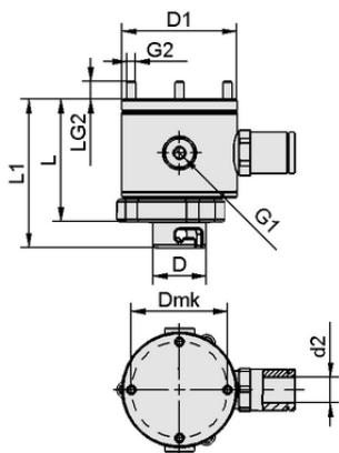
设计参数 VEE-RU 55x73.5 20 QCM
