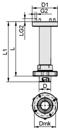
设计参数 VEE-FE 25.4x181.5
