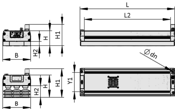
设计参数 FA-Xb SVK 1234 3R18 O20
