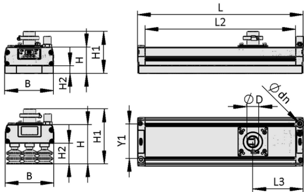
设计参数 FA-Mi SVK 442 3R18 O20
