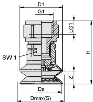
设计参数 SAXB 20 ED-85 G3/8-IG
