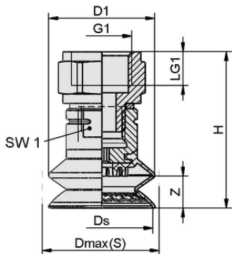
设计参数 SAXB 30 ED-85 G3/8-IG
